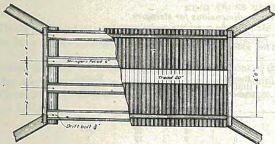
Plan Fig. 38
